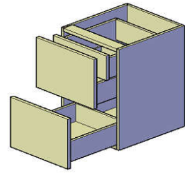
ARMÁRIO INFERIOR COM DUAS GAVETAS EXTERNAS E UMA INTERNA
